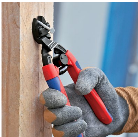
tête coudée à 20° avec couvre-joint d'un côté et coupante latérale pour une coupe nette; laisse de la place à la main pour saisir
